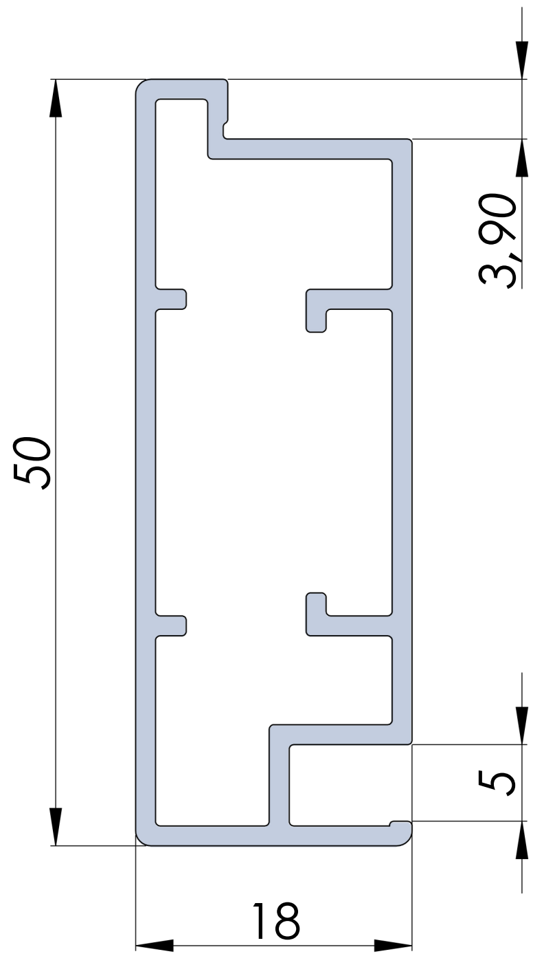
L1759 PERFIL A550 ESTANTE DOBLE VIDRIO
